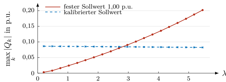
Abbildung 6.17: Maximaler Blindleistungsbetrag über \lambda für n = 40 und 10 % PV-Anteil. Bei kalibriertem Sollwert ist \max_k |Q_k| konstruktionsbedingt nahezu \lambda -invariant, bei festem Sollwert wächst er etwa mit \lambda^{1,3} .
