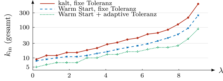
Abbildung 6.17: Gesamtzahl innerer Iterationen über \lambda für n = 40 und 10 % PV-Anteil, logarithmische Ordinate. Der Abstand der Kurven wächst mit dem Lastfaktor.
