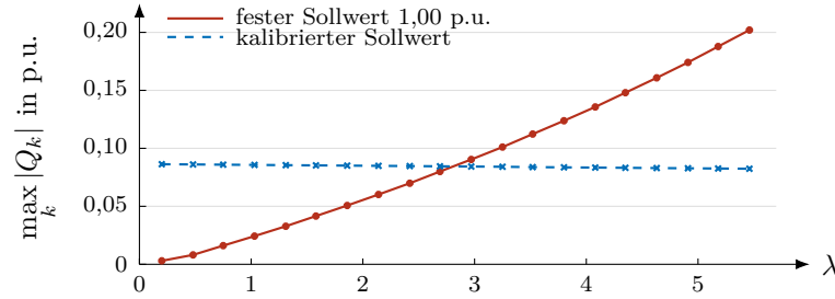
Abbildung 6.16: Maximaler Blindleistungsbetrag über \lambda für n = 40 und 10 % PV-Anteil. Bei kalibriertem Sollwert ist \max_k |Q_k| konstruktionsbedingt nahezu \lambda -invariant, bei festem Sollwert wächst er etwa mit \lambda^{1,3} .
