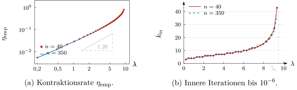
Abbildung 6.14: Innere Fixpunktiteration über dem Lastfaktor. Die Kurven für n = 40 und n = 350 liegen in (a) praktisch aufeinander; die gestrichelte Referenz kennzeichnet die Steigung 1,26 im Log-Log-Maßstab.
