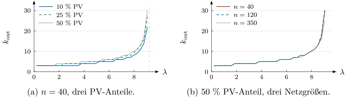
Abbildung 6.15: Äußere Iterationen der Blindleistungskorrektur bei kalibrierten Sollwerten. Die gestrichelte Vertikale in (a) markiert \lambda_{TPF}^* \approx 9,2 ; jenseits davon konvergiert kein Lauf.
