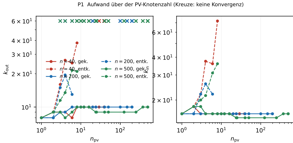
Abbildung 6.9: Äußere und gesamte innere Iterationen über der Zahl der PV-Knoten für n_{\text{bus}} \in \{40, 200, 500\} . Die gekoppelte Korrektur bildet ein Plateau; zum Vergleich ist die Abbruchkante der entkoppelten Variante eingezeichnet.
