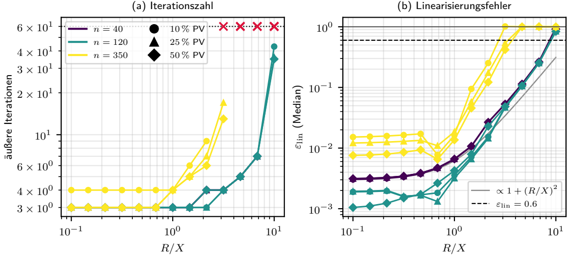
Abbildung 6.13: Äußere Q-Schleife im Modus const_z , gekoppelte Variante. Links die Zahl der äußeren Iterationen, rechts der relative Linearisierungsfehler \varepsilon_{\text{lin}} der Sensitivitätsbeziehung (Median über die äußeren Schritte) über \rho . Farbe kodiert die Netzgröße, der Marker den PV-Anteil. Rote Kreuze markieren Läufe ohne Konvergenz innerhalb von 60 äußeren Iterationen, die graue Linie im rechten Diagramm die Referenzsteigung \propto \rho^2 nach Gl. (6.9). Kernaussage: Plateau bis \rho \approx 1 bei drei Iterationen, danach Anstieg gemeinsam mit \varepsilon_{\text{lin}} .
