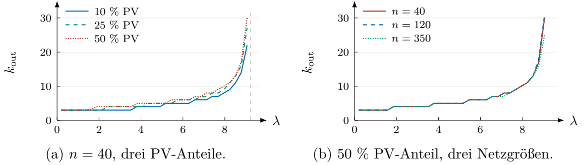
Abbildung 6.15: Äußere Iterationen der Blindleistungskorrektur bei kalibrierten Sollwerten. Die gestrichelte Vertikale in (a) markiert \lambda_{\text{TPF}}^* \approx 9,2 ; jenseits davon konvergiert kein Lauf.
