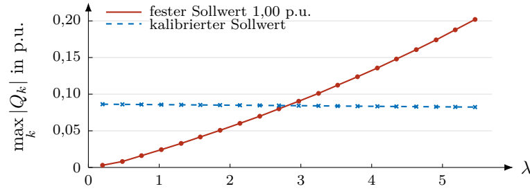
Abbildung 6.16: Maximaler Blindleistungsbetrag über \lambda für n = 40 und 10 % PV-Anteil. Bei kalibriertem Sollwert ist \max_k |Q_k| konstruktionsbedingt nahezu \lambda -invariant, bei festem Sollwert wächst er etwa mit \lambda^{1,3} .
