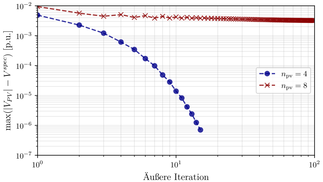
Abbildung 6.1: Konvergenzverhalten eines 40 Knoten Netzes mit n_{pv} = 4 und n_{pv} = 8 PV Knoten. Abgebildet wird der maximale Spannungsfehler des Verteilernetzes gegen die Iterationsschritte der äußeren Q-Korrektur.
