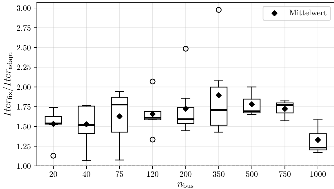
Abbildung 6.7: Einsparung der Iterationen Iter_{\text{fix}}/Iter_{\text{adapt}} der adaptiven inneren Toleranz gegenüber der fixierten Toleranz, aufgetragen über der Netzgröße n_{\text{bus}} . Jeder Boxplot fasst die Ergebnisse mehrerer PV-Anteile derselben Netzgröße zusammen. Die Box umfasst den Interquartilsabstand, die horizontale Linie den Median, die Raute den Mittelwert, die Whisker den 1,5-fachen Interquartilsabstand und die Kreise die außerhalb liegenden Einzelkonfigurationen.
