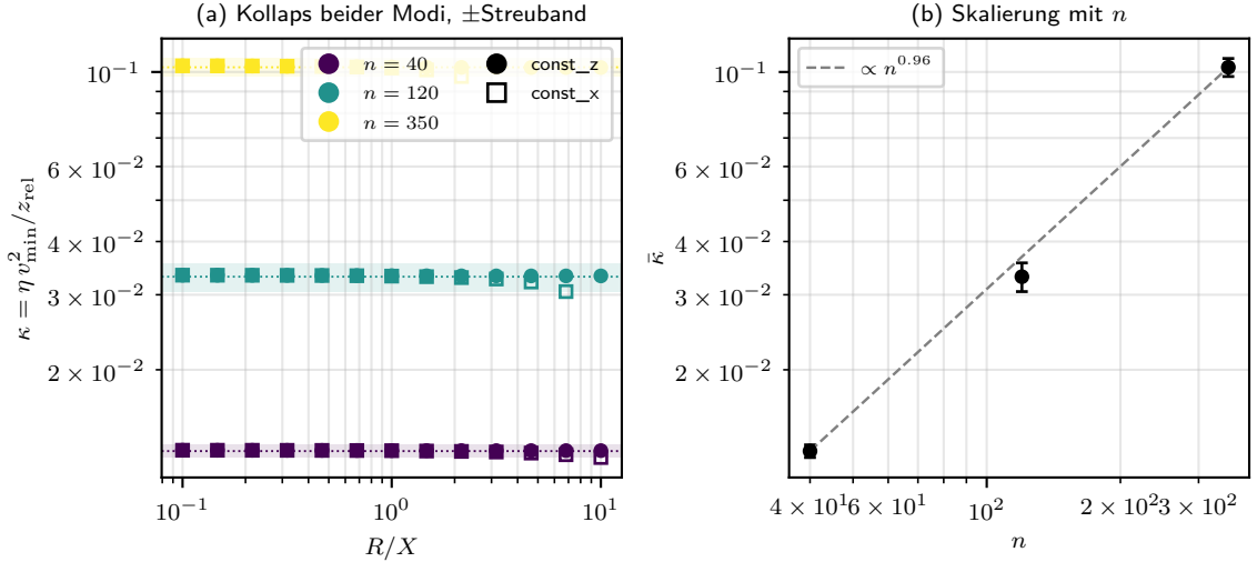
Abbildung 6.13: Test der Skalierung (6.9) ( n_{\text{pv}} = 0 ). (a) Rohdaten wie in Abbildung 6.12, hier mit an Diagramm (b) angepasster Achsenskalierung: const_z (durchgezogen, gefüllte Kreise) verläuft flach, const_x (gestrichelt, offene Quadrate) entlang der grauen Referenz \propto \sqrt{1 + \rho^2} . (b) Nach Reskalierung fallen beide Modi je Netzgröße auf einen konstanten Wert zusammen; die Restschwankung bleibt unter 3,4 %. Die Netzgröße wird nicht wegskaliert, die drei Niveaus bleiben getrennt.
