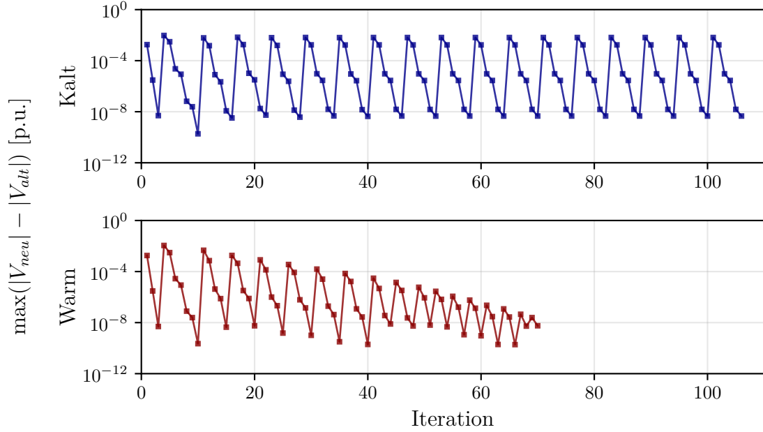
Abbildung 6.5: Gesamtiterationsverlauf für ein 40-Knoten-Netz mit n_{pv} = 4 PV-Knoten bei Cold Start (oben) und Warm Start (unten). Abgebildet ist die Spannungsänderung \max(|V_{neu}| - |V_{alt}|) je innerer Iteration über alle äußeren Iterationen hinweg.
