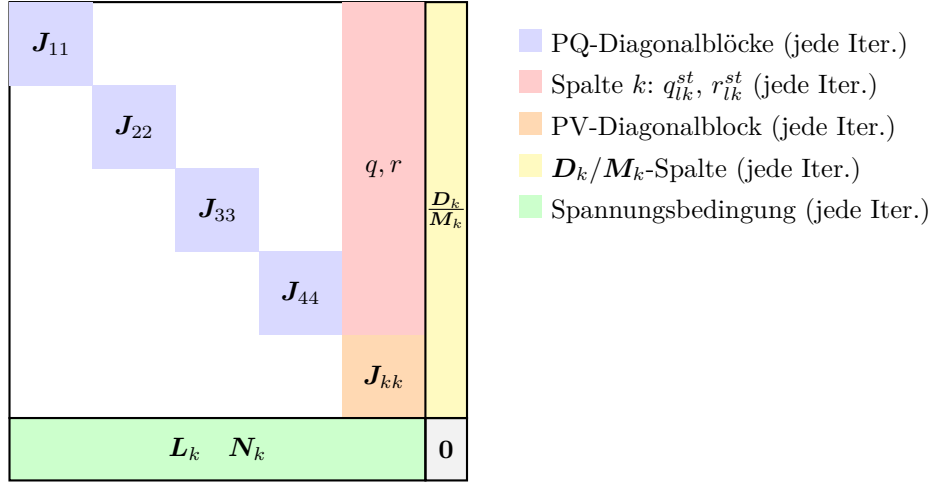
Abbildung 1.1: Schematische Struktur der erweiterten Jacobi-Matrix mit PV-Knoten gemäß [4]. Die Außerdiagonalblöcke der PQ-Knoten (weiß) sind konstant. Die gesamte Spalte des PV-Knotens sowie die zusätzliche \Delta Q -Spalte und Spannungsbedingungszeile müssen in jeder Iteration aktualisiert werden.
