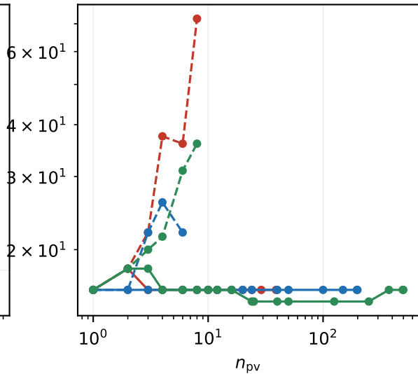
P1 Aufwand über der PV-Knotenzahl (Kreuze: keine Konvergenz)
