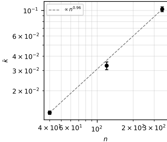
(b) Skalierung mit n
