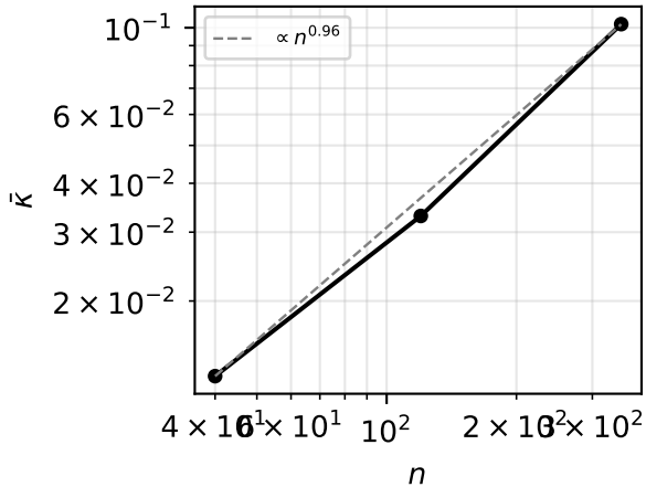
(b) Skalierung mit n
