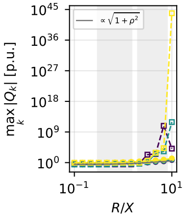
(a) Q-Bedarf
