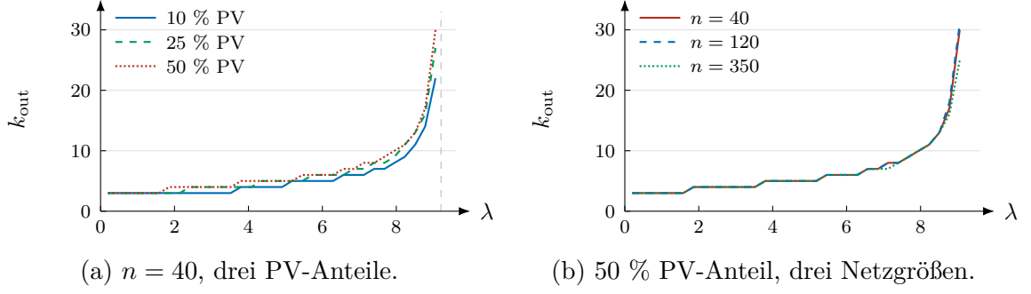
Abbildung 6.16: Äußere Iterationen der Blindleistungskorrektur bei kalibrierten Sollwerten. Die gestrichelte Vertikale in (a) markiert \lambda_{TPF}^* \approx 9,2 ; jenseits davon konvergiert kein Lauf.
