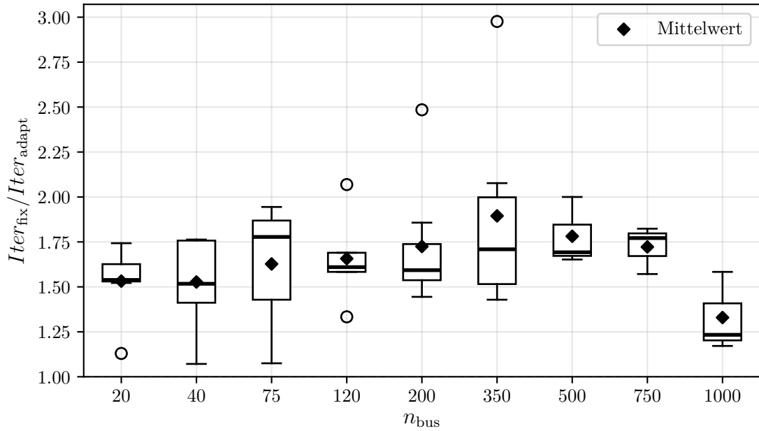
Abbildung 6.7: Einsparung der Iterationen \text{Iter}_{\text{fix}}/\text{Iter}_{\text{adapt}} der adaptiven inneren Toleranz gegenüber der fixierten Toleranz, aufgetragen über der Netzgröße n_{\text{bus}} . Jeder Boxplot fasst die Ergebnisse mehrerer PV-Anteile derselben Netzgröße zusammen. Die Box umfasst den Interquartilsabstand, die horizontale Linie den Median, die Raute den Mittelwert, die Whisker den 1,5-fachen Interquartilsabstand und die Kreise die außerhalb liegenden Einzelkonfigurationen.
