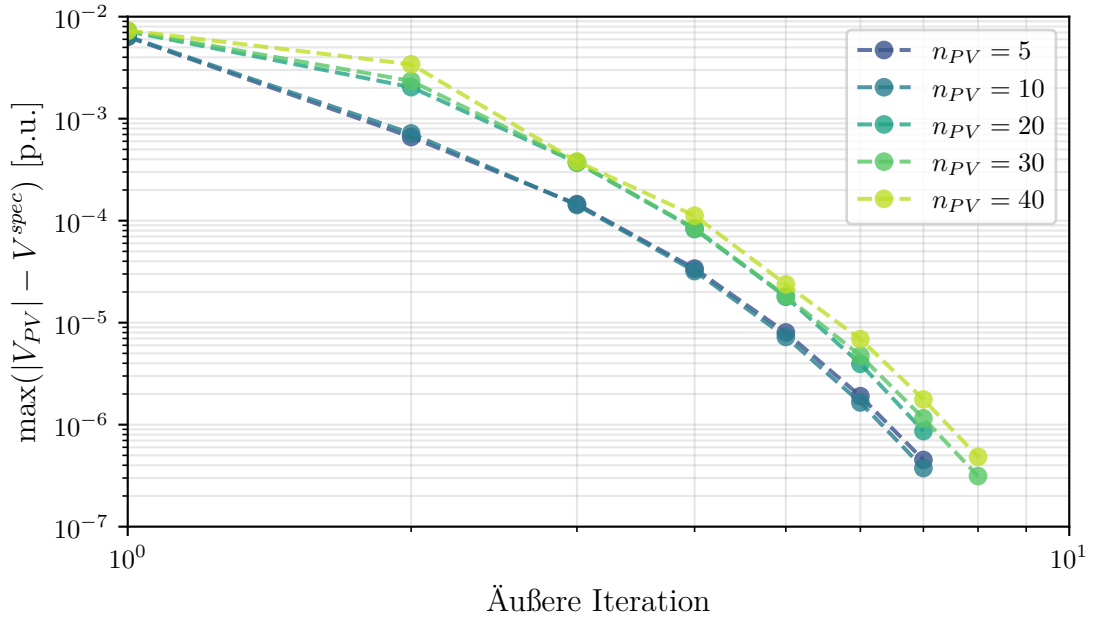
Abbildung 6.4: Konvergenzverhalten der gekoppelten Q-Korrektur für das 40-Knoten-Netz bei n_{pv} \in \{5, 10, 20, 30, 40\} PV-Knoten. Abgebildet wird der maximale Spannungsfehler gegen die Iterationsschritte der äußeren Q-Korrektur.
