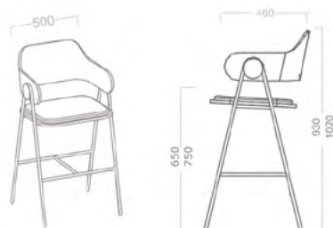
BANQUETA BIA (fixa)
