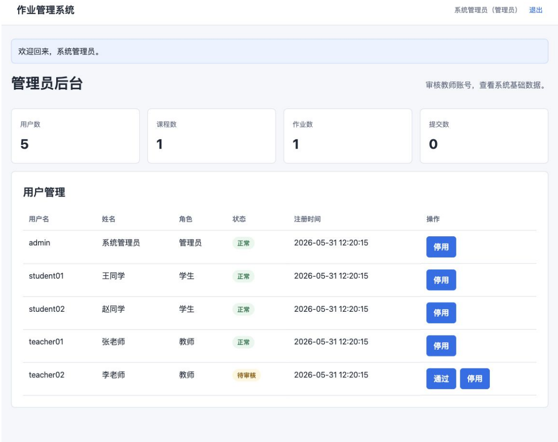
图 9: 管理员后台
