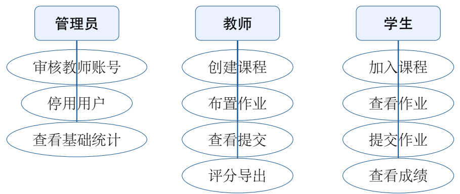
图 3: 系统用例图
