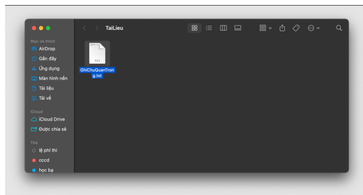
Bước 8
