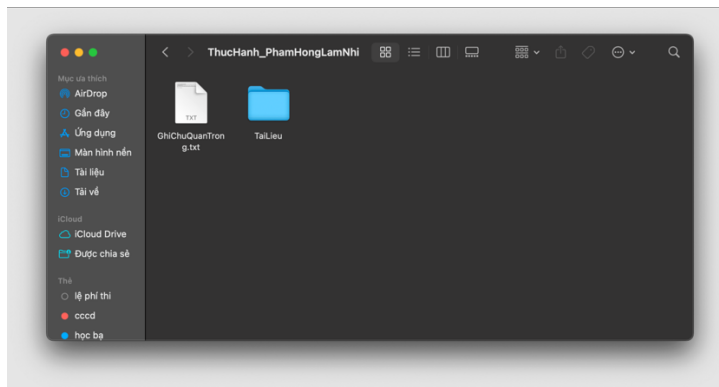
Bước 7
