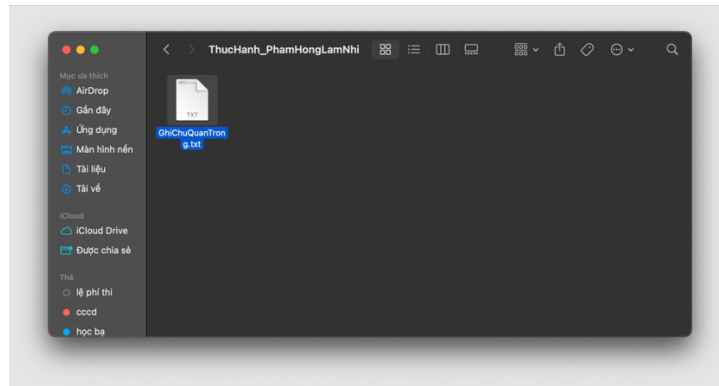
Bước 6
