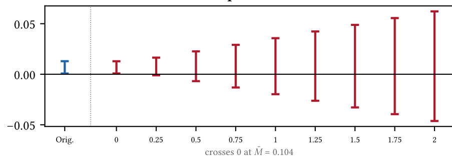
Spillover
