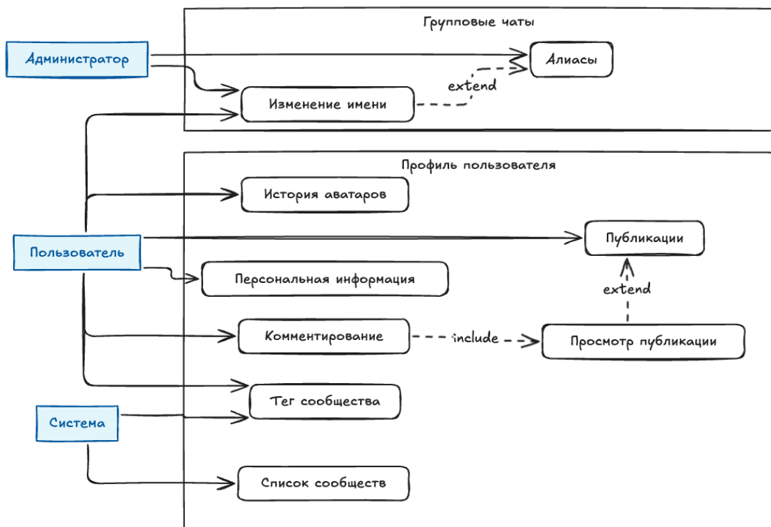
Рисунок 3 — Диаграмма прецедентов
