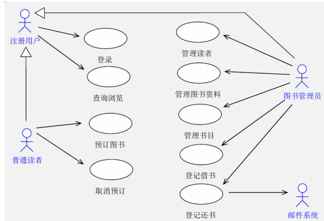
图 1 MiniLibrary 系统用例图
