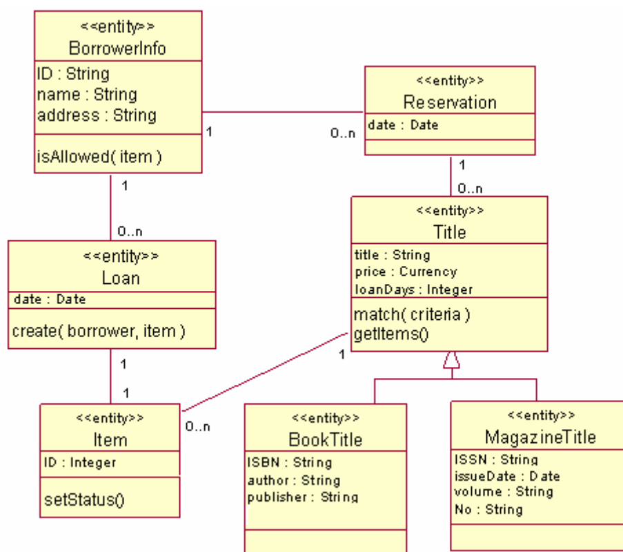
图 2 实体类类图
