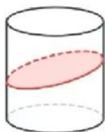
椭圆
