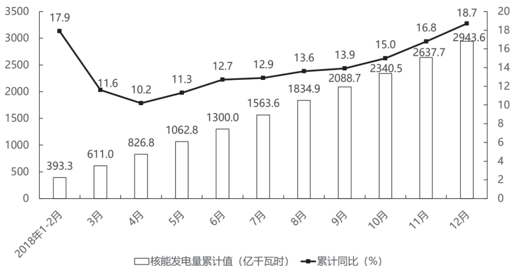
2018 年 1~12 月某国核能发电量统计及增长情况
