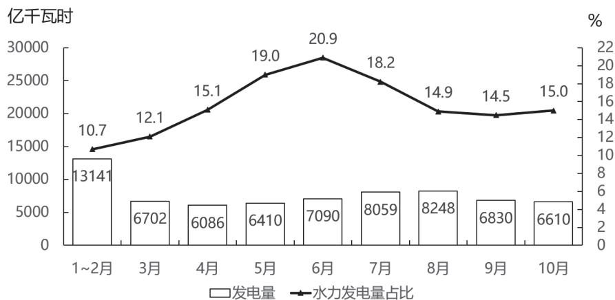
2022年1~10月H国发电量及水力发电量占发电量比重
