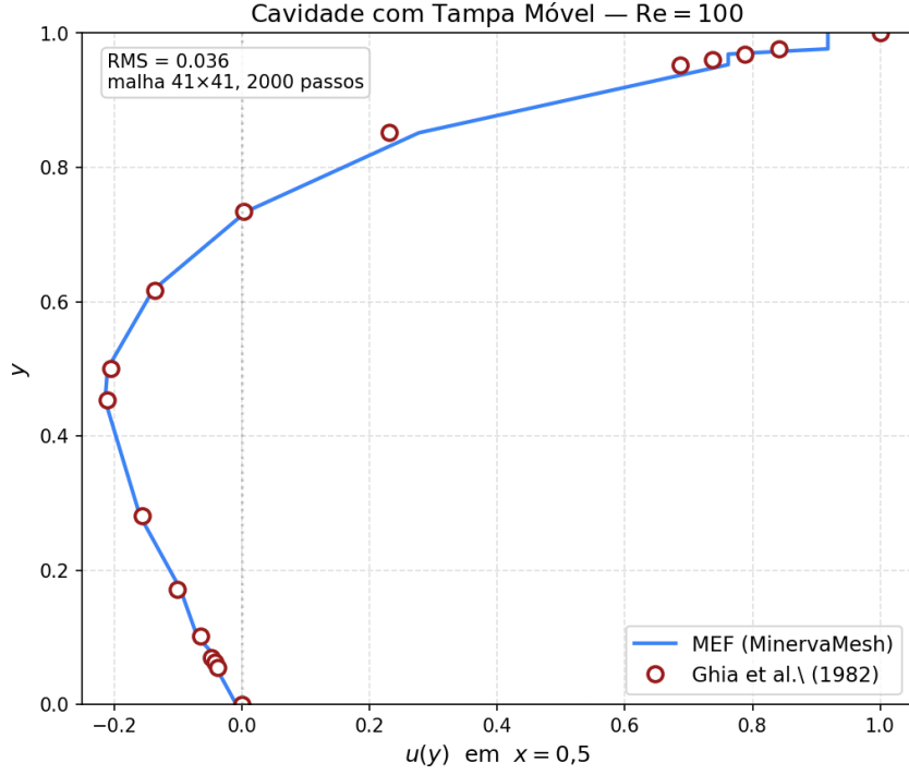
Figura 6.10: Perfil u(y) em x = 0,5 comparado aos valores tabulados por Ghia et al. [31] para a cavidade com tampa móvel a Re = 100 . RMS = 0,036 em malha 41 \times 41 com 2000 passos de tempo.
