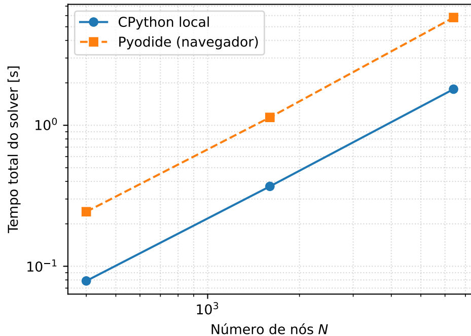
Transcador 2D MEF (esparso, 50 passos)
