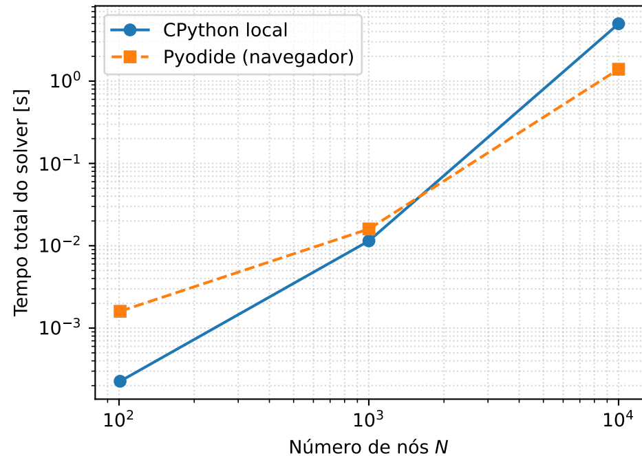
Condução 1D MEF (denso)
