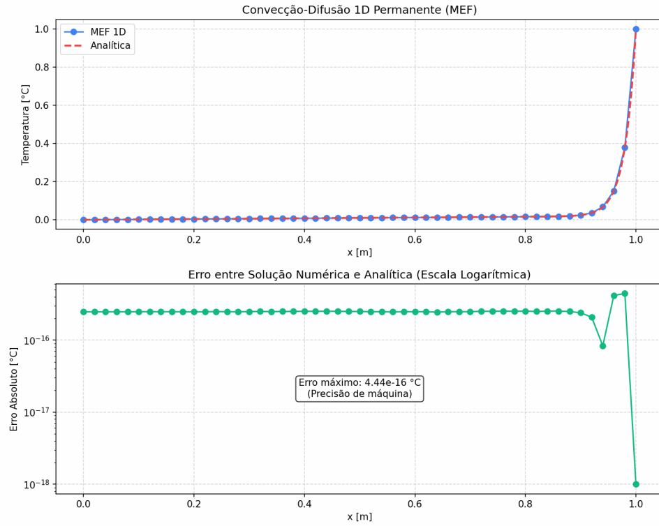
Figura 6.3: Convecção-difusão 1D com SUPG ativo em Pe_e = 0,5 . Painel superior: temperatura T(x) — pontos azuis para o MEF e linha tracejada vermelha para a solução analítica, visualmente coincidentes em toda a malha. Painel inferior: erro absoluto |T^{\text{MEF}} - T^{\text{ana}}| em escala logarítmica, com máximo 4,44 \times 10^{-16} \text{ }^{\circ}\text{C} — precisão de máquina.
