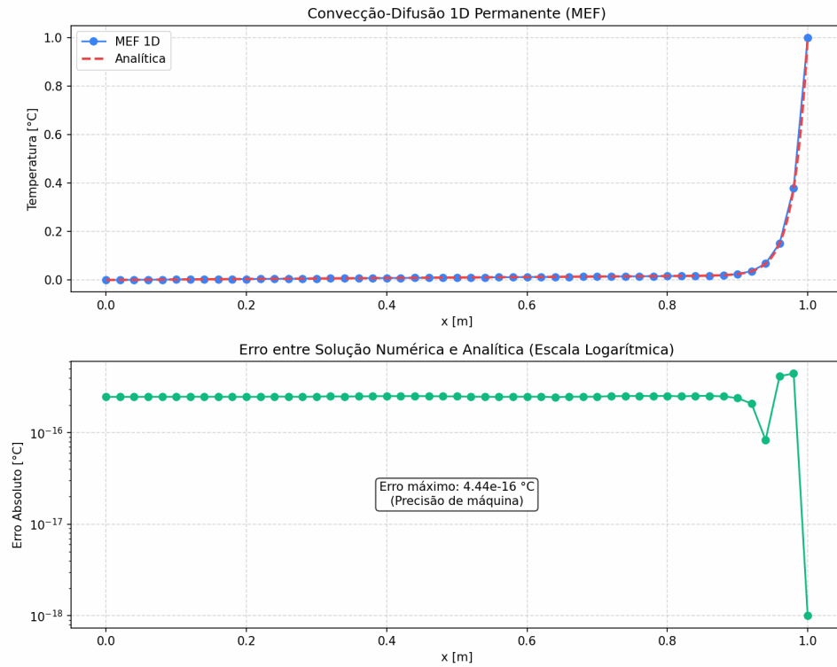
Figura 5.3: Convecção-difusão 1D com SUPG ativo em Pe_e = 0,5 . Painel superior: temperatura T(x) — pontos azuis para o MEF e linha tracejada vermelha para a solução analítica, visualmente coincidentes em toda a malha. Painel inferior: erro absoluto |T^{\text{MEF}} - T^{\text{ana}}| em escala logarítmica, com máximo 4,44 \times 10^{-16} °C — precisão de máquina.
