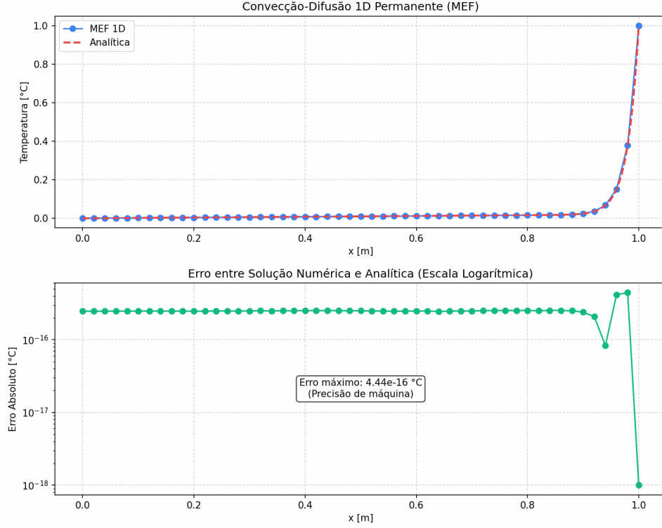
Figura 6.3: Convecção-difusão 1D com SUPG ativo em \text{Pe}_e = 0,5 . Painel superior: temperatura T(x) — pontos azuis para o MEF e linha tracejada vermelha para a solução analítica, visualmente coincidentes em toda a malha. Painel inferior: erro absoluto |T^{\text{MEF}} - T^{\text{ana}}| em escala logarítmica, com máximo 4,44 \times 10^{-16} \text{ °C} — precisão de máquina.
