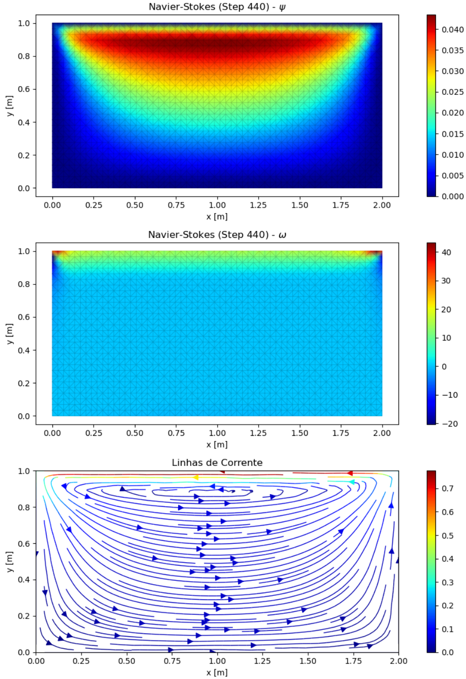
Figura 5.8: Navier-Stokes 2D — cavidade com tampa móvel ( Re = 100 ): campos de \psi , \omega e linhas de corrente.
