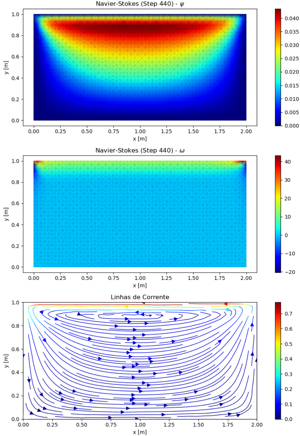
Figura 4.10: Navier-Stokes 2D — cavidade com tampa móvel ( Re = 100 ): campos de \psi , \omega e linhas de corrente.
