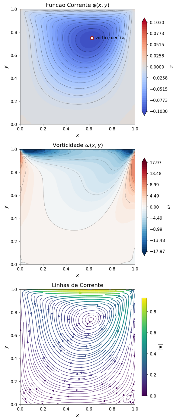
Figura 5.8: Cavidade com tampa móvel a Re = 100 : função de corrente \psi (topo), vorticidade \omega (meio) e linhas de corrente sobre o campo de magnitude de velocidade (base). O vórtice primário está centrado em (0,625; 0,750) com \psi_{\min} = -0,103 . A intensa vorticidade negativa sob a tampa é a assinatura da camada-limite induzida pelo cisalhamento.
