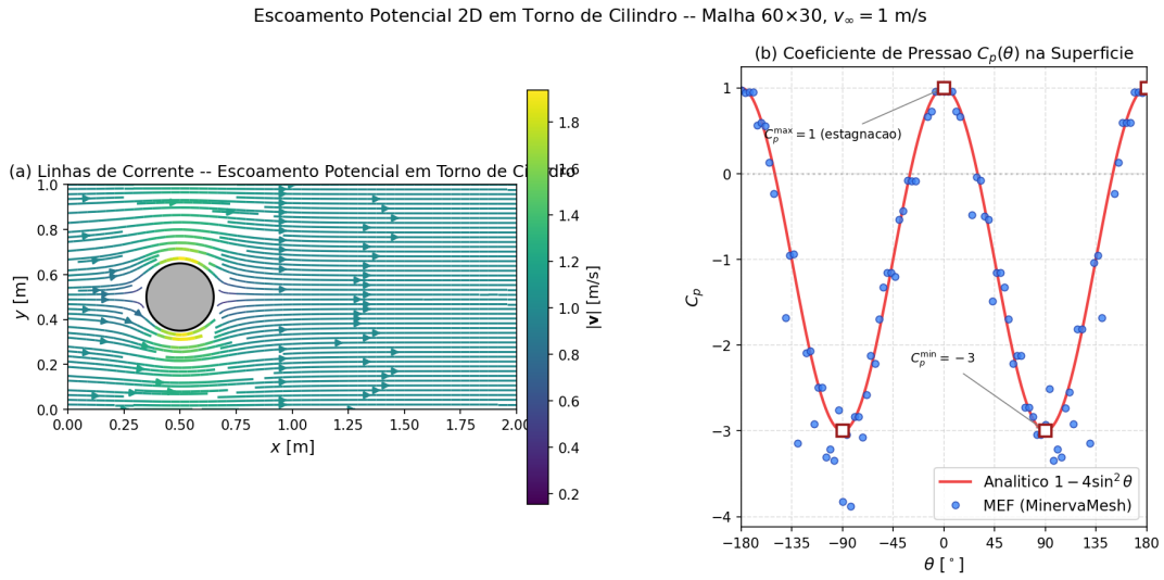
Figura 5.7: Escoamento potencial em torno de cilindro: linhas de corrente (esquerda) e distribuição de C_p(\theta) sobre a superfície (direita). A simulação (azul) reproduz a estrutura qualitativa do escoamento simétrico, com os pontos de estagnação frontal/traseiro e os polos de pressão mínima próximos dos valores teóricos C_p = 1 e C_p = -3 . A quebra de simetria entre \theta = +90^\circ e \theta = -90^\circ é consequência do confinamento lateral do domínio ( 2r/H = 30\% ) e do viés da malha estruturada.
