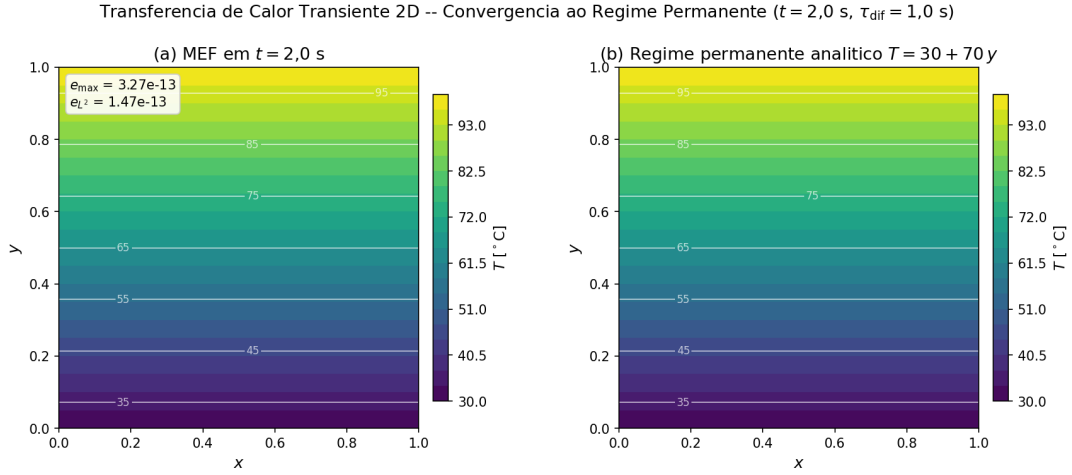
Figura 5.6: Transferência de calor transiente 2D: campo T(x, y) MEF em t = 2,0 s (esquerda) comparado ao perfil analítico de regime permanente T_{\infty}(x, y) = 30 + 70y (direita). As isothermas MEF são horizontais, confirmando a invariância em x prevista pela solução analítica.
