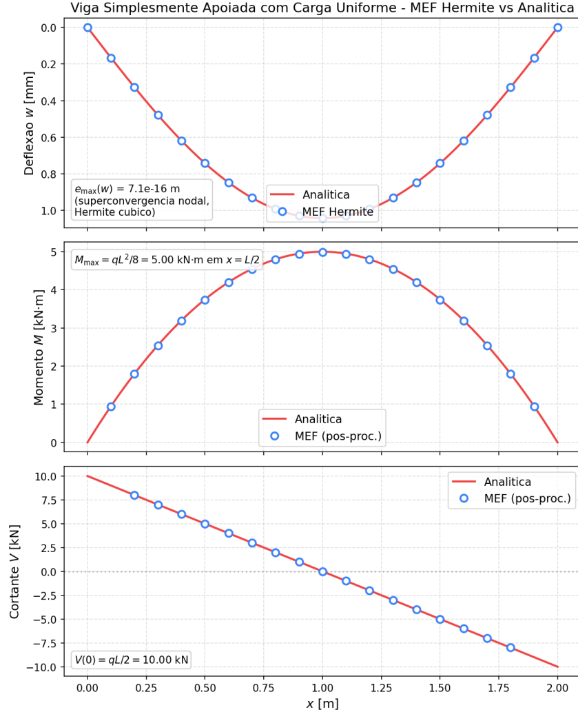
Figura 5.4: Viga simplesmente apoiada com carga uniforme: deflexão w(x) (topo), momento fletor M(x) (meio) e esforço cortante V(x) (base). Pontos azuis representam a solução MEF com elementos de Hermite cúbicos; linha vermelha, a solução analítica. A deflexão máxima MEF coincide com w_{\max} = 5qL^4/(384EI) = 1,0417 mm; M e V são reconstruídos por diferenciação numérica da deflexão nodal, o que explica o leve ruído próximo aos apoios (pontos de borda omitidos).
