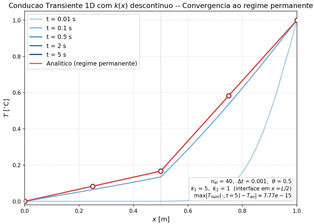
Figura 5.2: Condução transiente 1D com condutividade descontínua ( k_1 = 5 , k_2 = 1 ): evolução temporal do campo T(x, t) (curvas em azul, alpha crescente com o tempo) comparada à solução analítica de regime permanente (linha sólida vermelha). A malha de 40 elementos P1 com \theta = 1/2 reproduz fielmente o kink de condutividade em x = L/2 e converge para T(L/2) = 1/6 .
