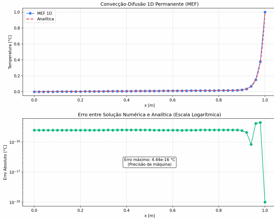
Figura 4.3: Convecção-difusão 1D com SUPG ativo em \text{Pe}_e = 0,5 . Painel superior: temperatura T(x) — pontos azuis para o MEF e linha tracejada vermelha para a solução analítica, visualmente coincidentes em toda a malha. Painel inferior: erro absoluto |T^{\text{MEF}} - T^{\text{ana}}| em escala logarítmica, com máximo 4,44 \times 10^{-16} \text{ °C} — precisão de máquina.
