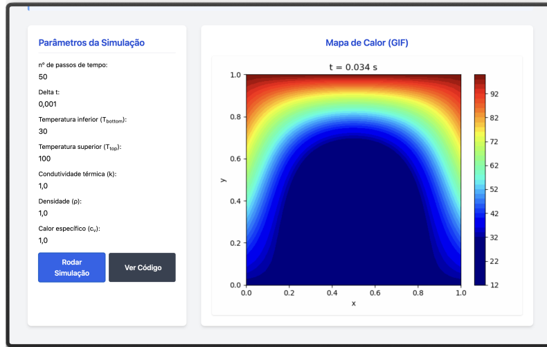
Figura 5.9: Campo de temperatura em placa 2D durante a evolução transiente (método de Crank-Nicolson).
