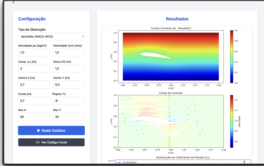
Figura 5.10: Escoamento potencial 2D: linhas de corrente ao redor de um obstáculo.
