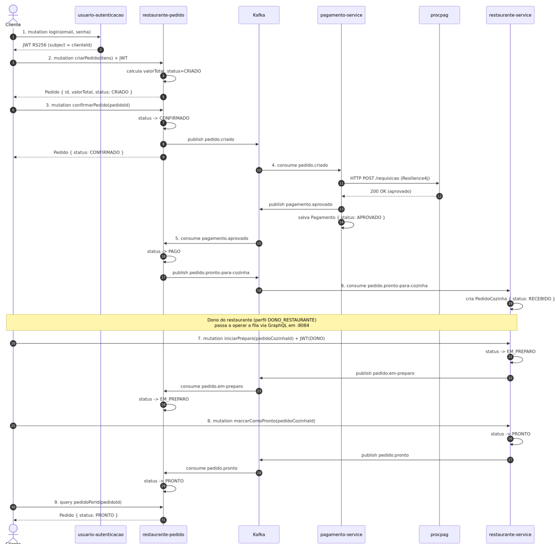
Figura 2 — Sequência do fluxo feliz (cadastro → entrega pela cozinha).
