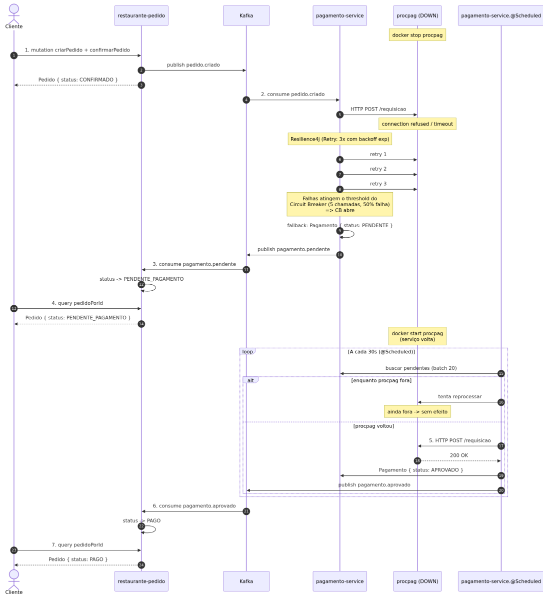
Figura 3 — Sequência de falha do gateway + reprocessamento automático.
