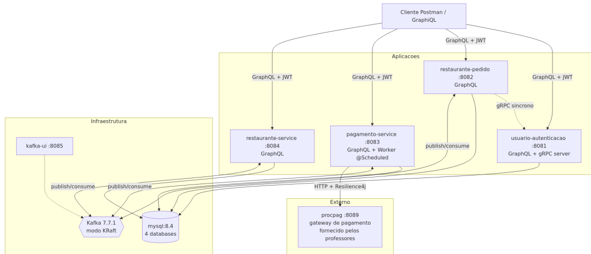
Figura 1 — Diagrama de componentes do sistema.
