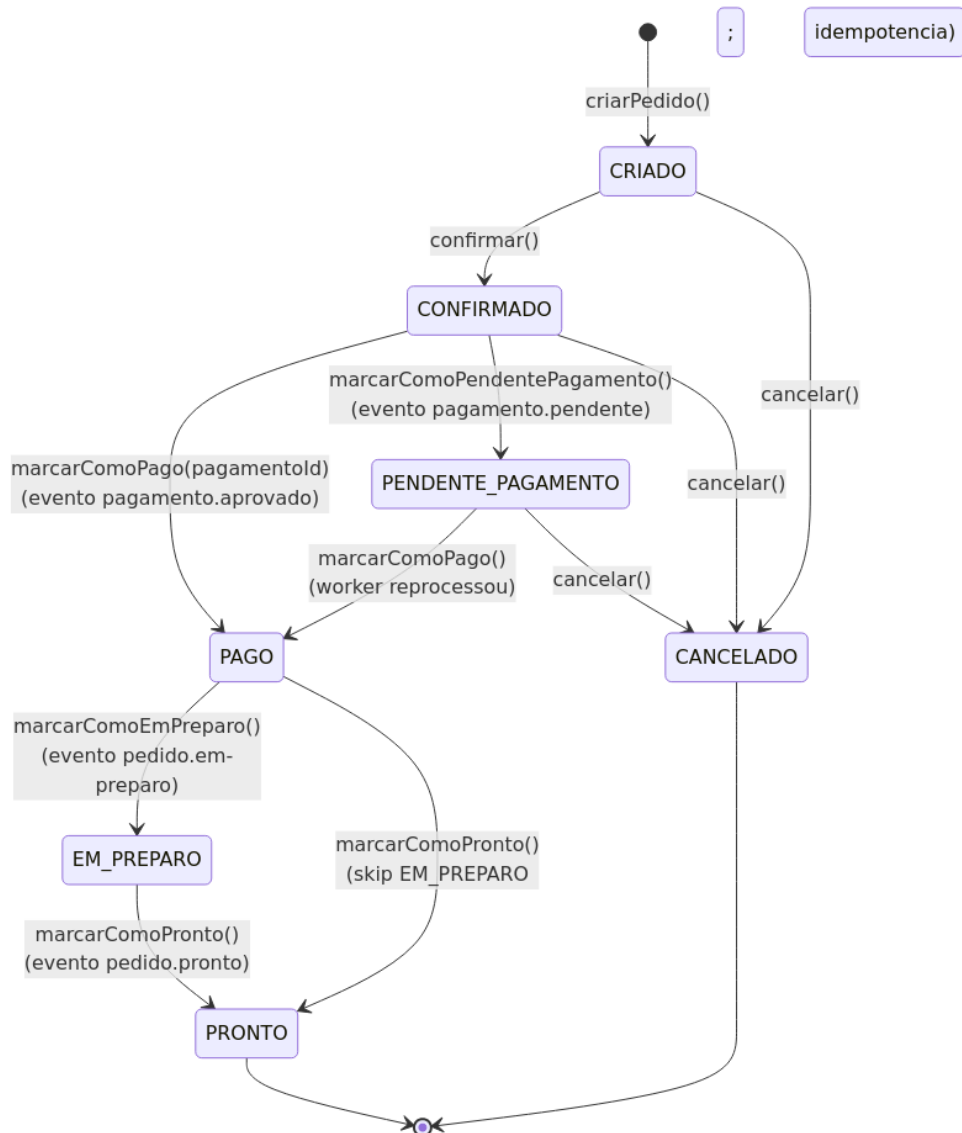
Figura 4 — Máquina de estados do agregado Pedido.
