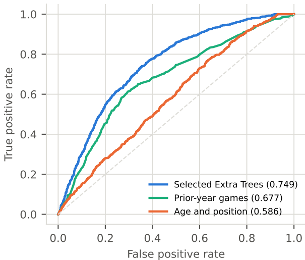
ROC, 2022-2024 audit
