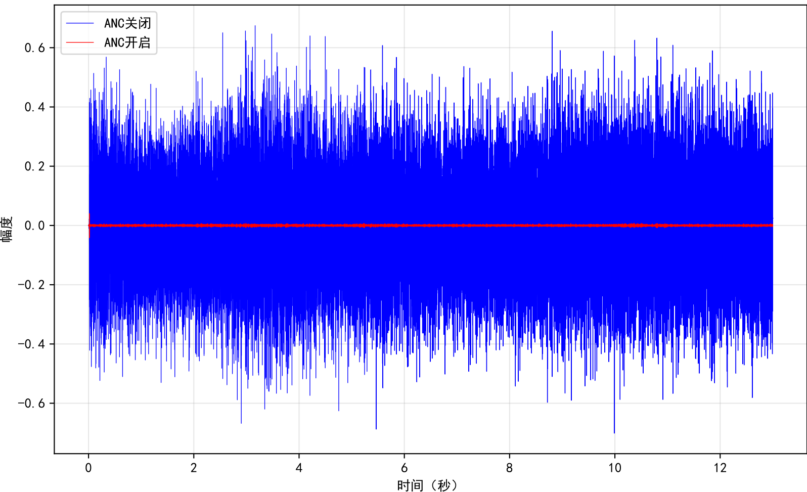
SFANC-FxNLMS混合算法性能对比
