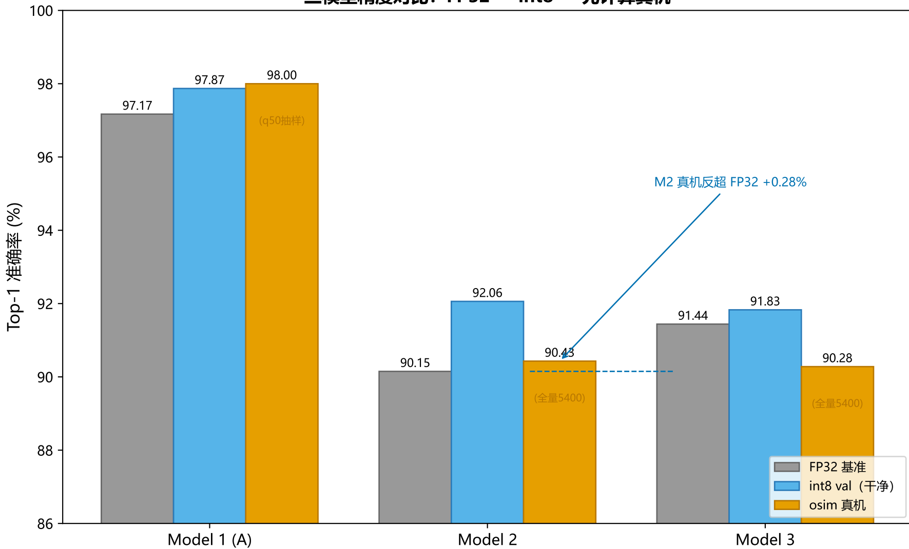
三模型精度对比: FP32 → int8 → 光计算真机
