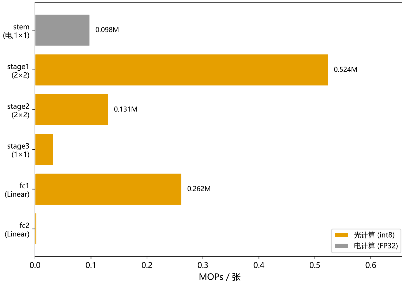
逐层运算量分布 (补零浪费 = 0)
