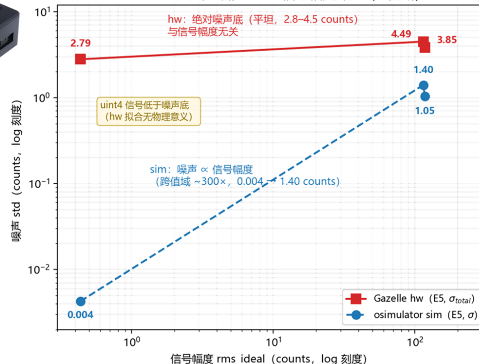
E5: hw 绝对噪声底 vs sim 信号相关噪声 (3 值域)
