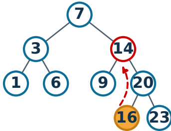
2) Nachfolger: 16
