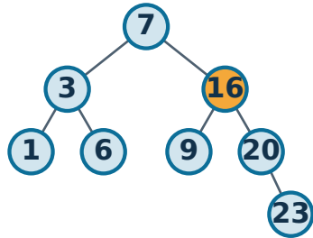
3) 16 ersetzt 14
