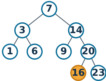
1) 16 einfügen
