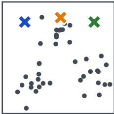
1) Init (K=3)
