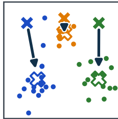
3) Update
