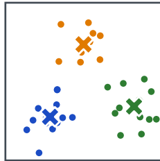
4) konvergiert
