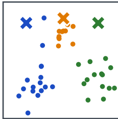
2) Assign
