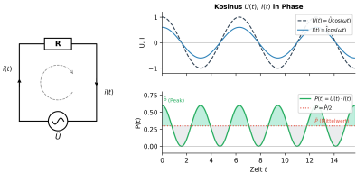
Am ohmschen Widerstand: U und I in Phase, P \geq 0
