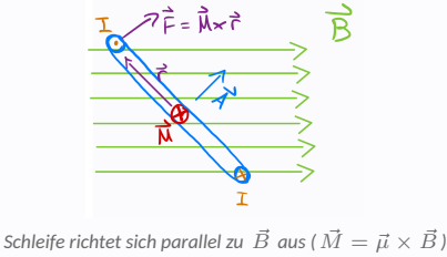
Schleife richtet sich parallel zu \vec{B} aus ( \vec{M} = \vec{\mu} \times \vec{B} )
