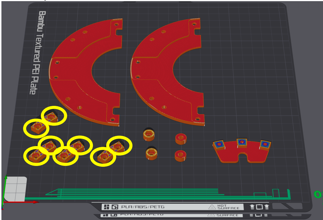
Pause 4, layer 41
