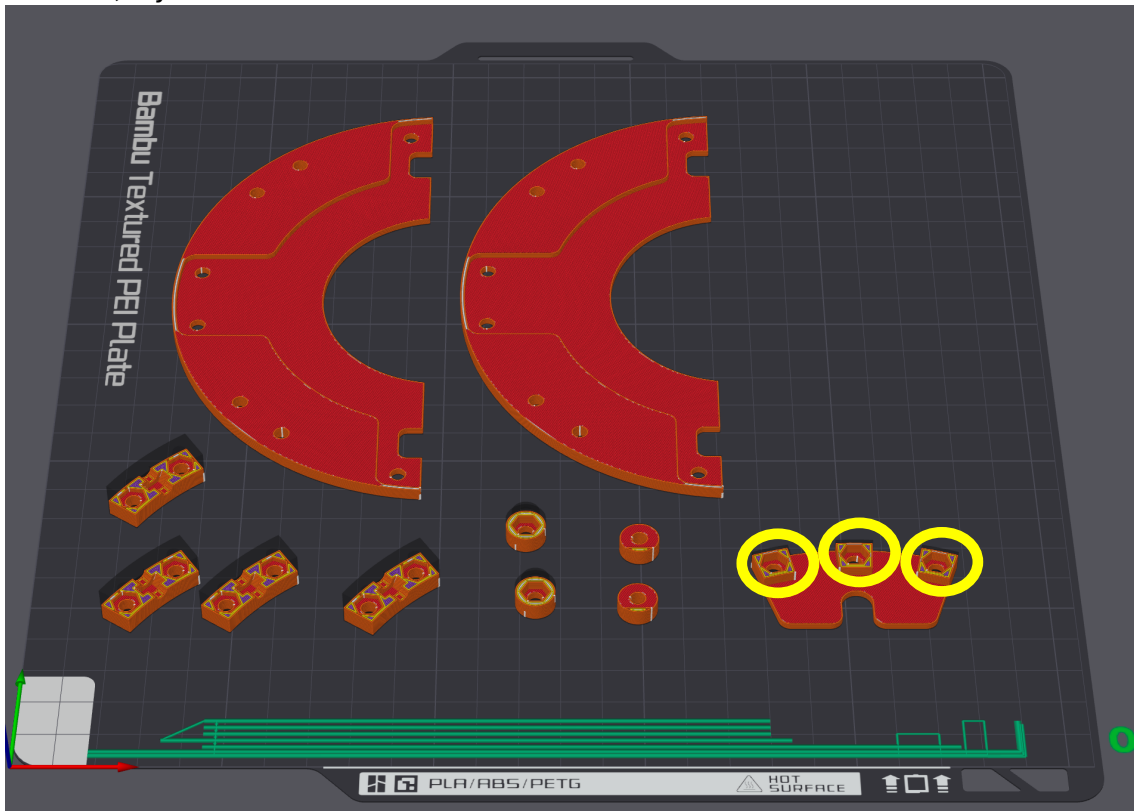
Pause 2, layer 26
