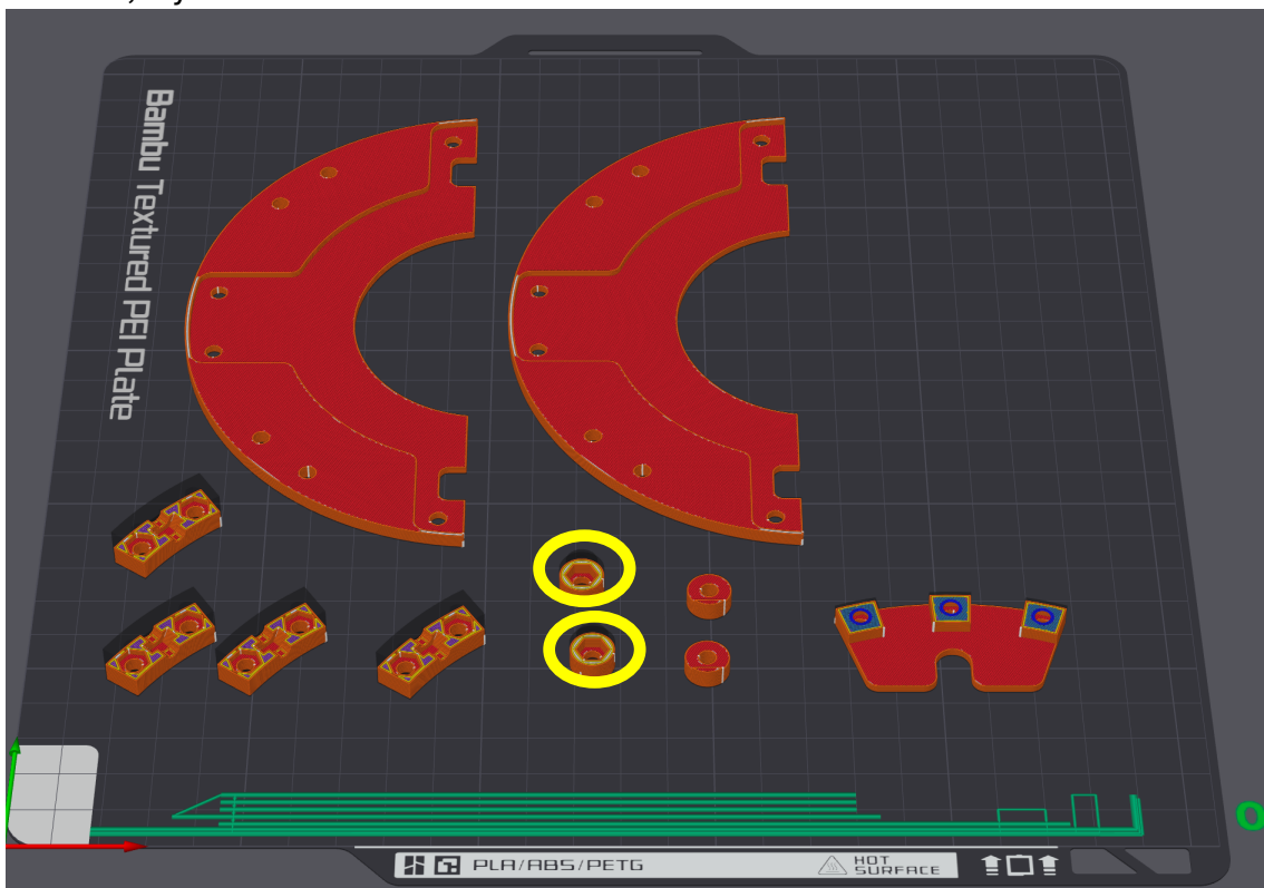
Pause 2, layer 26
