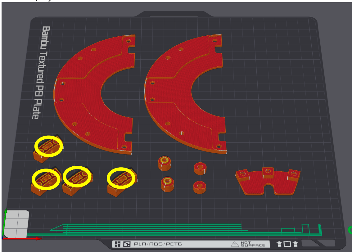
Pause 4, layer 41
