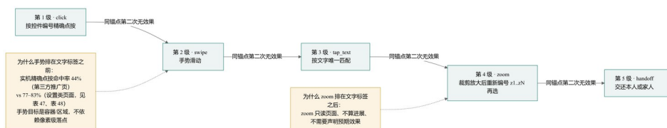
图 7 有界升级阶梯：click → swipe → tap_text → zoom → handoff 与排序依据
