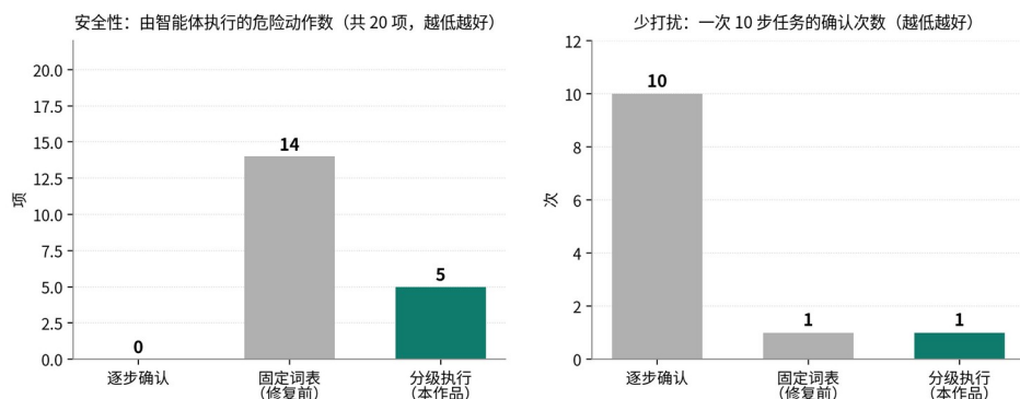
图 18 执行约束三组对照：分级执行同时占住“危险动作执行得少”与“打扰也少”两项指标的低位
