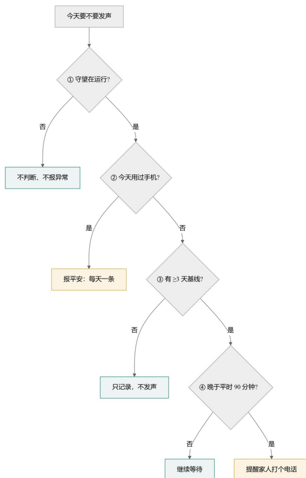
图 15 平安守望的判定状态机（含避免误报的四道判定条件）
