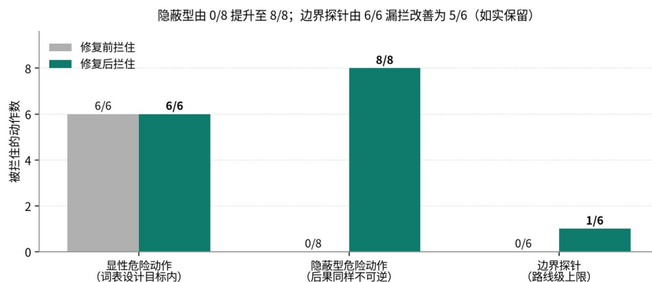
图 17 词表覆盖面：隐蔽型危险动作由 0/8 到 8/8，边界探针仍 5/6 漏拦
