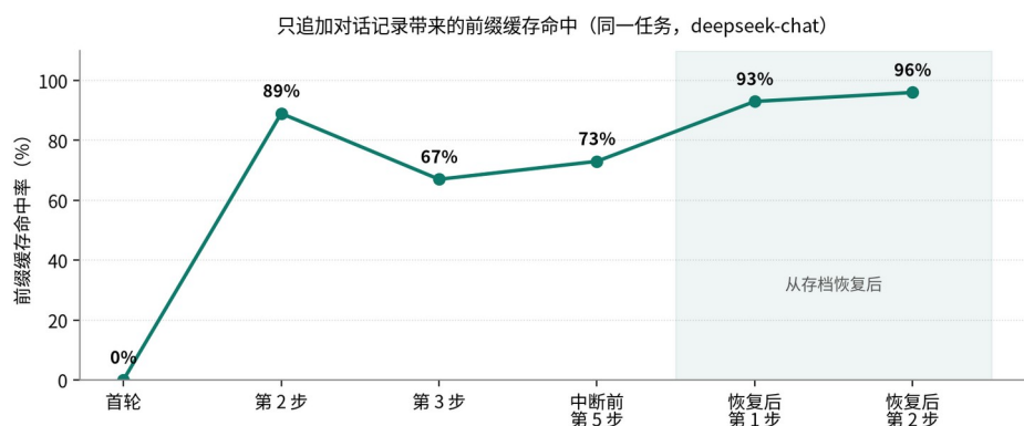
图 21 只追加对话记录带来的前缀缓存命中：改动系统指令前缀即失效，命中率随之跌落
