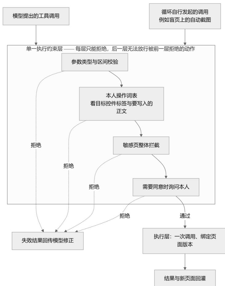
图 3 单一执行入口与单调执行约束层：模型发起的与循环自行发起的调用走同一层
