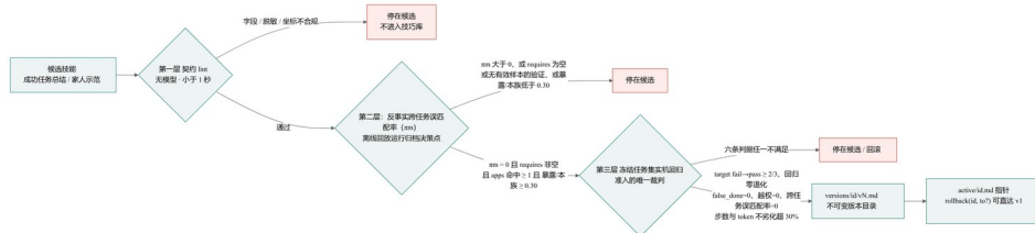
图 8 技能准入的三层判定：第一层契约 lint → 第二层反事实跨任务误匹配率 ( \pi m ) → 第三层冻结任务集实机回归 → 不可变版本与回滚
