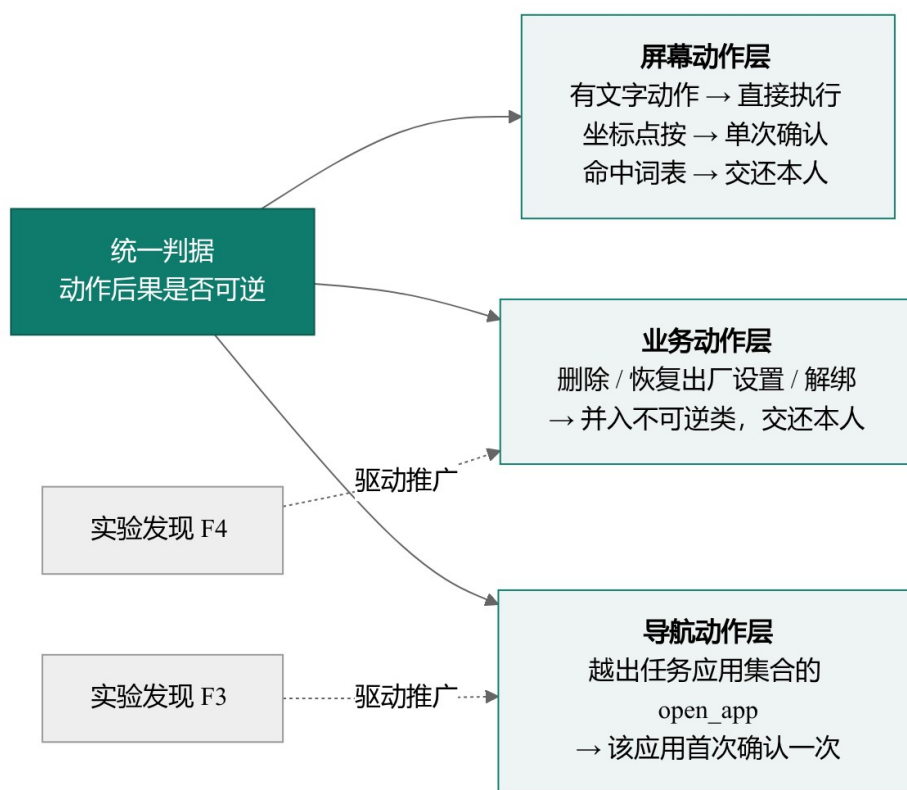
图 6 一个判据的三层复用：屏幕动作 / 业务动作 / 导航动作
