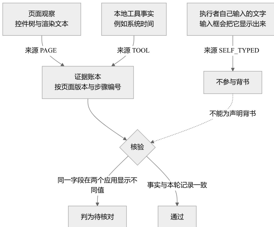
图 5 证据来源三分：哪一类事实可以为完成声明背书
