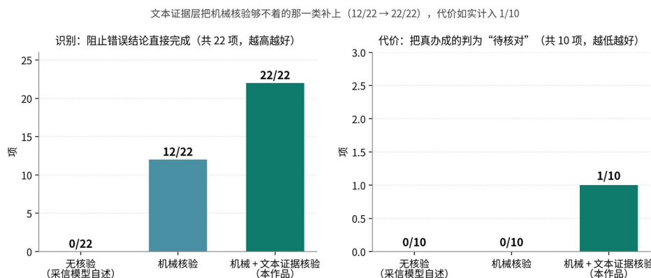
图 19 完成核验的分层收益与代价：文本证据层把机械核验够不着的那一类补上（12/22 → 22/22），保守代价如实计入 1/10
