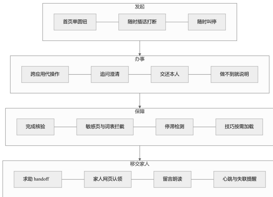
图 9 功能架构：发起 / 办事 / 保障 / 移交家人
