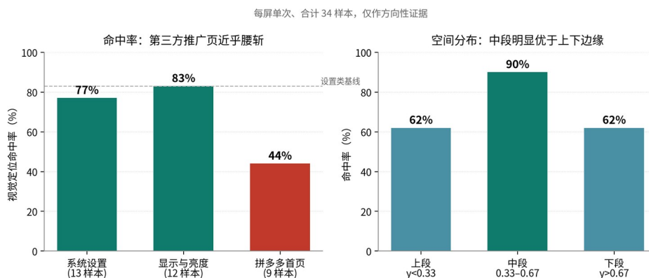
图 20 实机坐标定位的命中率与空间分布（每屏单次、合计 34 样本）
