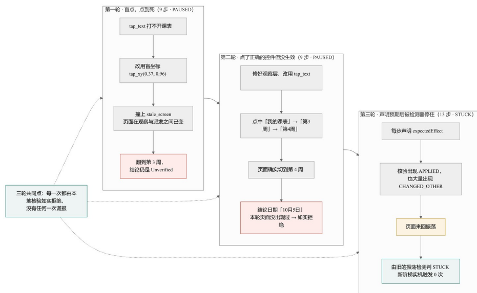
图 11 S1 查课表的三轮演进：盲点 → 点中正确控件 → 被检测器停住
