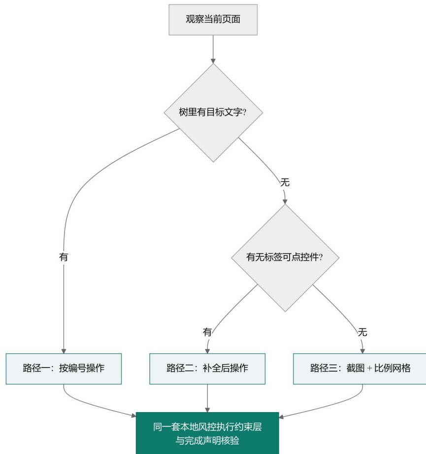
图 14 观察层的三条路径与自动切换
