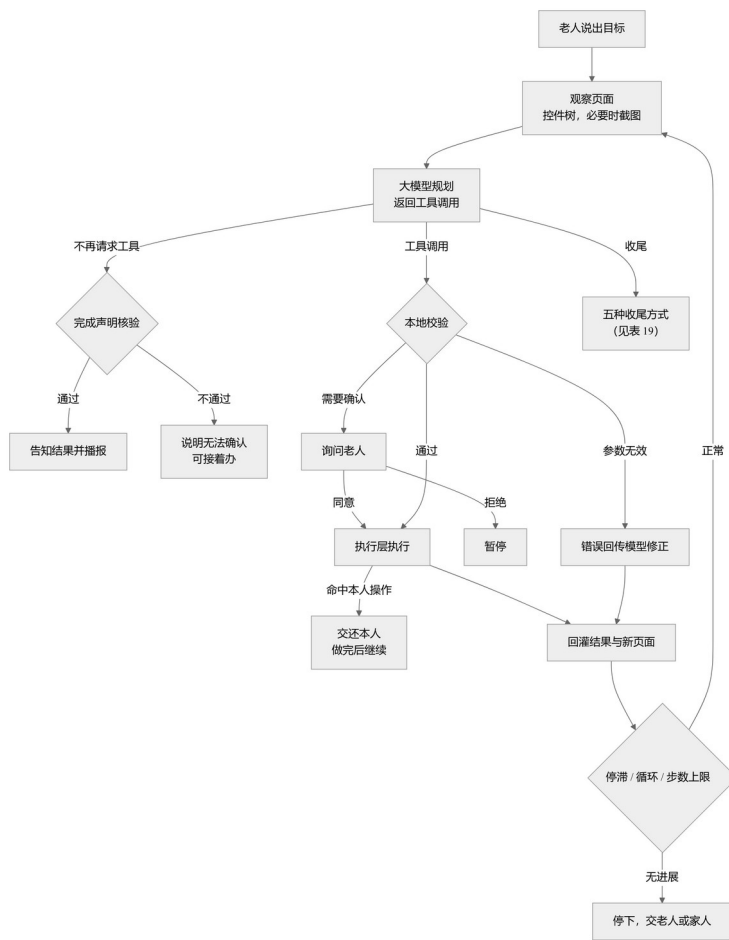
图 10 任务执行流程与五种收尾方式
