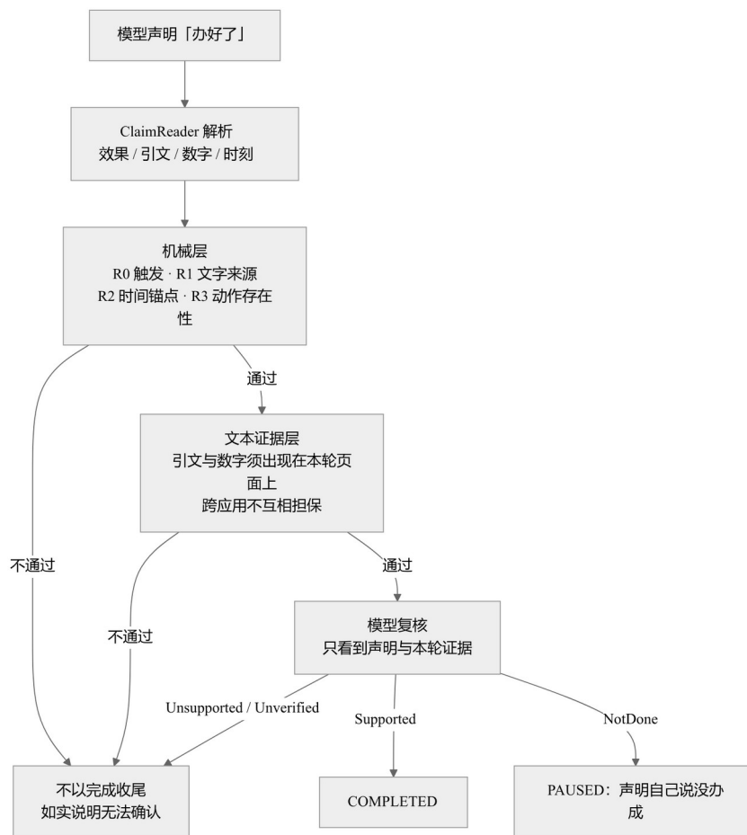
图 4 完成声明核验的两级串联：本机核验通过后才允许模型复核
