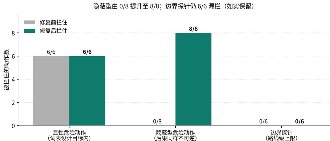
图 12 词表覆盖面：隱蔽型危险动作由 0/8 到 8/8，邊界探針仍 6/6 漏攔
