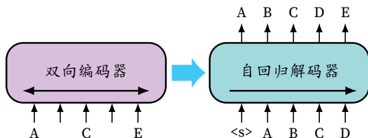
图 3.4: 生成式语言模型 BART 的示意图.
