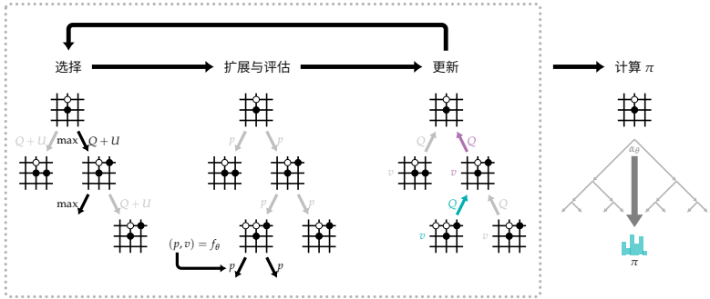
图 9.5: \text{MCTS} 的过程
