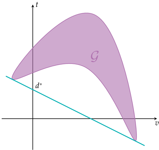
图 7.6: 对偶规划的最优值 d^*
