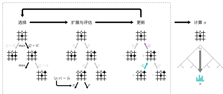
图 9.5: MCTS 的过程
