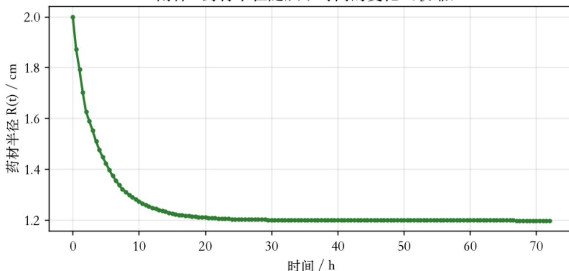
附件2 药材半径随烘干时间的变化（收缩）
