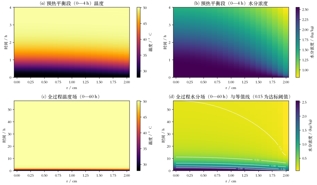
Figure 8: 问题 2/3 场图
