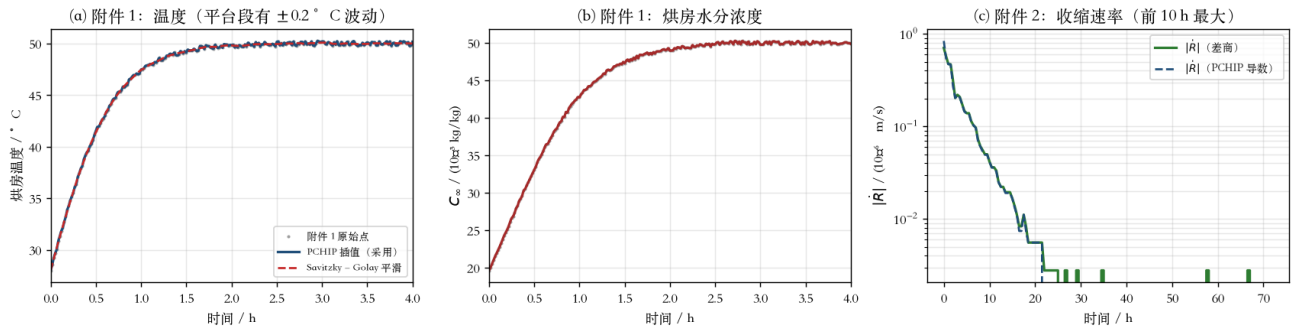
Figure 2: 数据图
