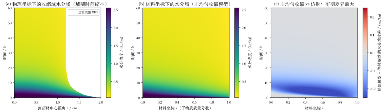
Figure 12: 问题 4 场图
