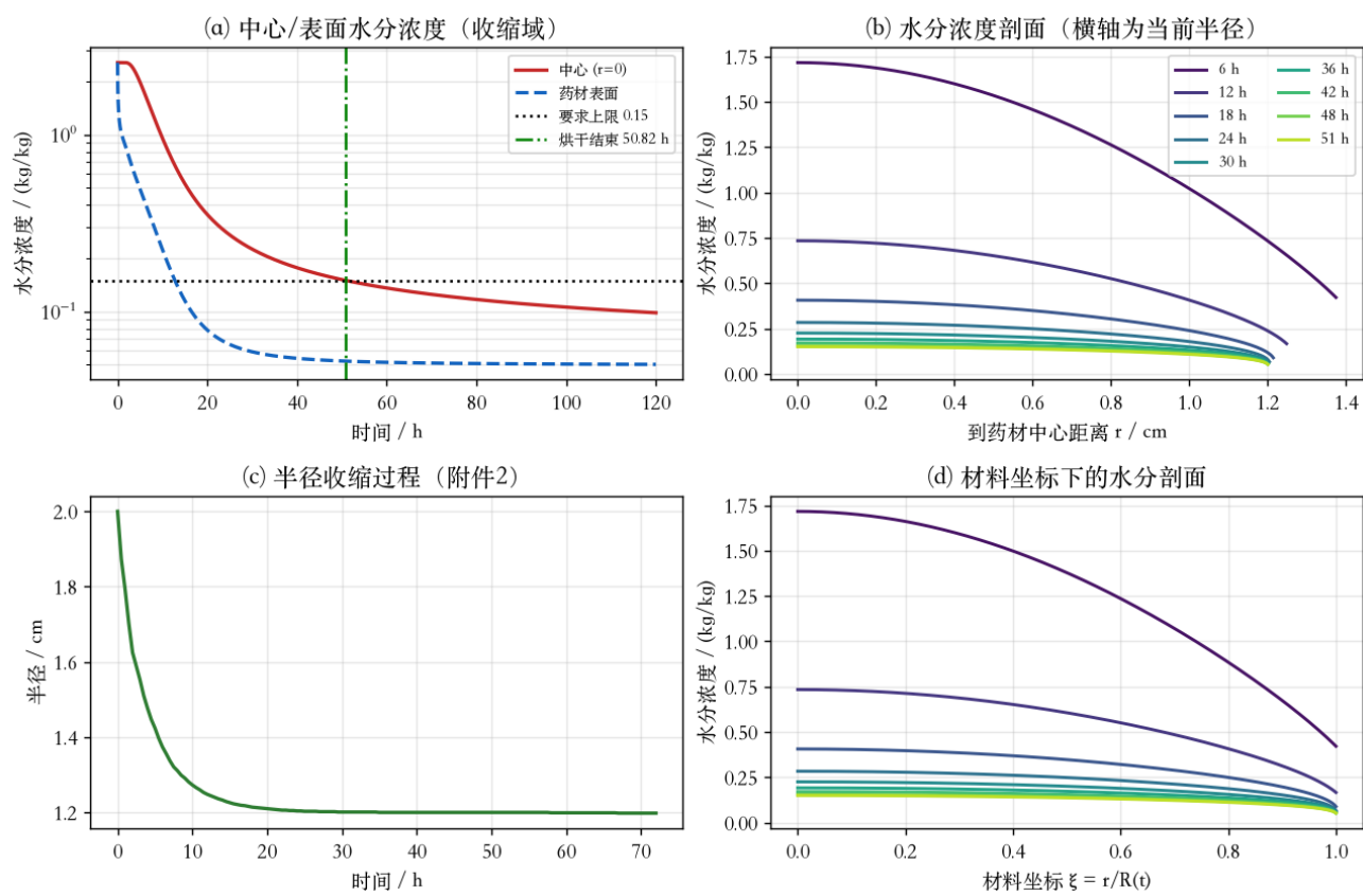
Figure 11: 问题 4 结果
