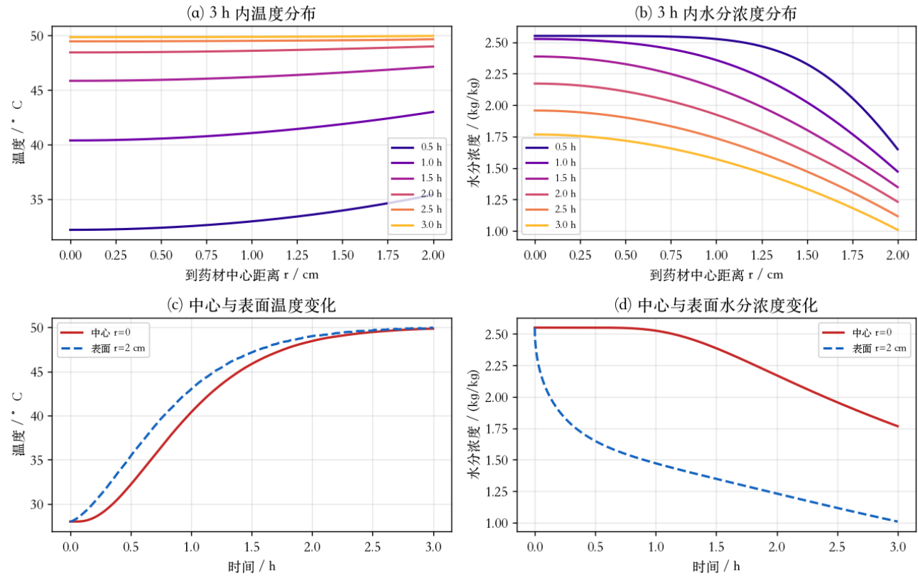
Figure 7: 问题 2 结果
