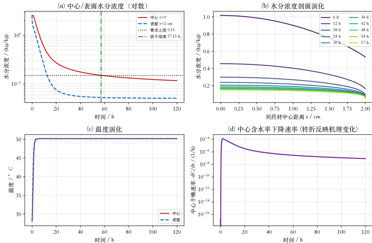
Figure 9: 问题 3 结果
