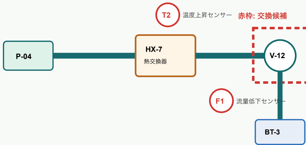
図1: 冷却ラインCL-2の異常箇所。赤枠はV-12バイパス弁を示す。T2温度上昇とF1流量低下が同時に出た場合、V-12固着を第一候補として点検する。
