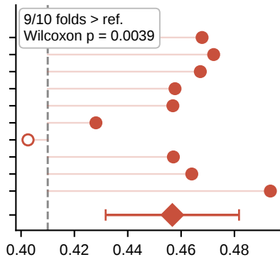
Boundary F1
