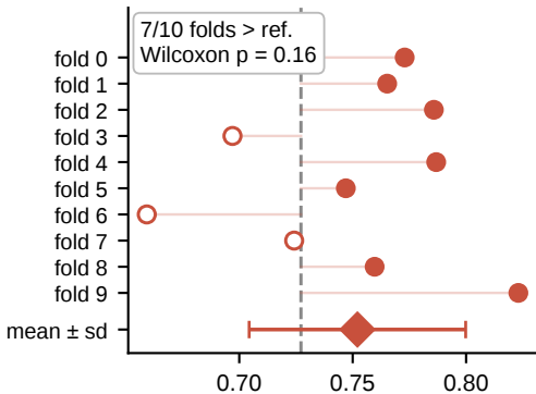
Weighted F1
