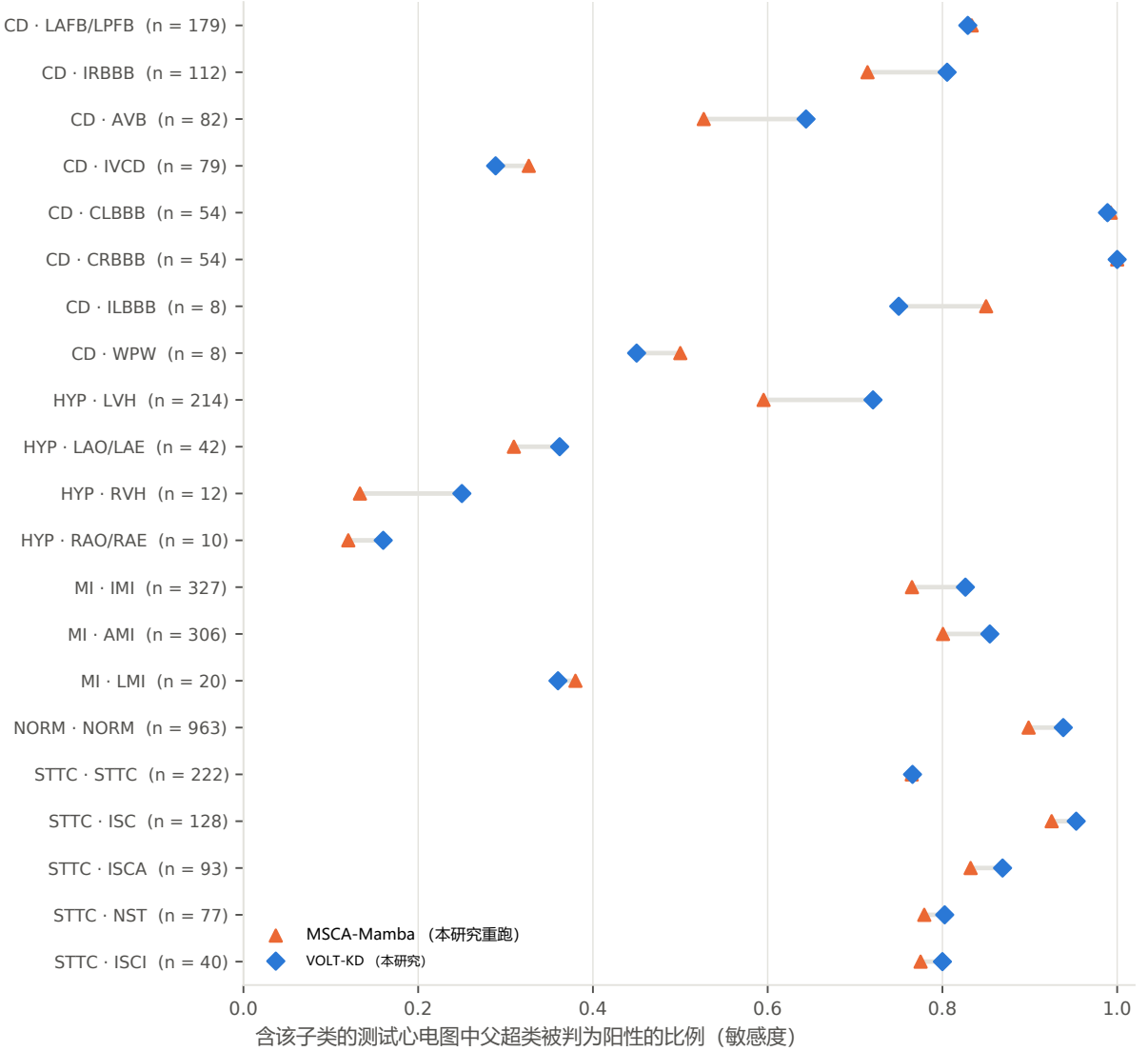
图 6: 完整 VOLT-KD 与本地 MSCA-Mamba 在各诊断子类记录中的父类检出比例。纳入至少五条测试记录的子类，数值和样本量见表 S4。
