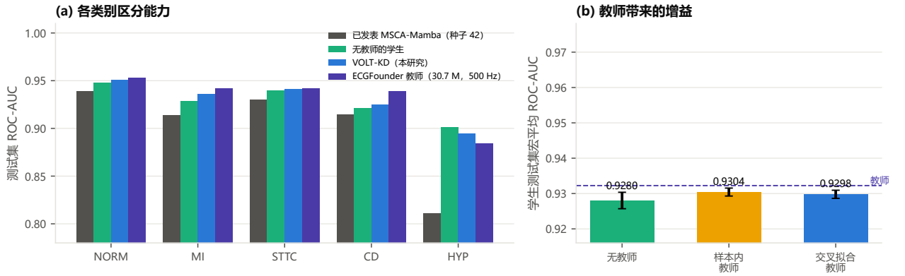
图 4: ECGFounder 教师与本文 VOLT-KD 学生的逐类及整体结果。教师为四个留出模型的测试集 logits 集成；学生为五种子均值；图内教师参数量按单个成员标注，集成总参数量见表 8；文献 MSCA-Mamba 为原文种子 42 参照。
