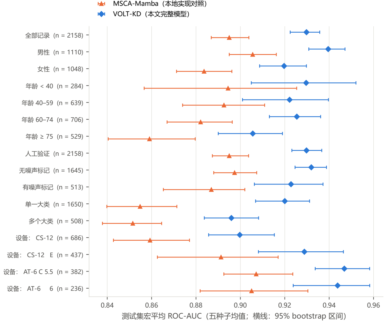
图 9: 本文完整 VOLT-KD 学生模型与本地 MSCA-Mamba 对照模型在不同测试亚组中的宏平均 ROC-AUC。蓝色菱形为完整 VOLT-KD, 橙色三角形为 MSCA-Mamba 本地实现; 点表示各模型五个种子的指标均值, 横向区间为各组内 300 次记录级 bootstrap 得到的 95% 区间。两种模型在同一测试折按人口、设备、质量和标签共现条件分组评价; 具体样本量和数值见表 S5。
