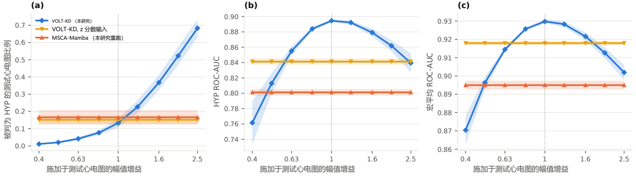
图 8: 完整 VOLT-KD、其 z-score 输入对照与本地 MSCA-Mamba 对全局电压增益的响应。相同测试波形乘以给定增益，模型参数、标签及验证阈值保持固定。
