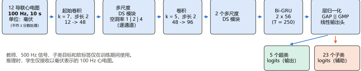
图 1: 幅值保留的训练与推理流程。高采样率记录、教师软标签和诊断子类只在训练阶段使用；推理阶段输入为 100 Hz 心电图，输出为五个诊断大类。完整 VOLT-KD 使用大类、子类与教师监督。
